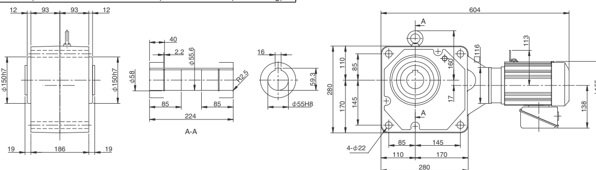
Fig. 5 RNYM08-1640-300~1440 Mass 68kg (RNYM08-1640-B-300~1440) (Mass 70kg)
