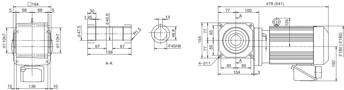
Fig. 2 RNYM3-1520-5~30 (RNYM3-1520-B-5~30) Mass 34kg (Mass 39kg)
