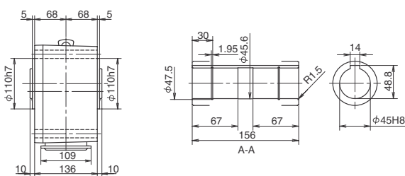
Fig. 5 RNYM05-1640-CB-300-1440 Mass 68kg (RNYM05-1640-CB-B-300-1440) (Mass 70kg)
