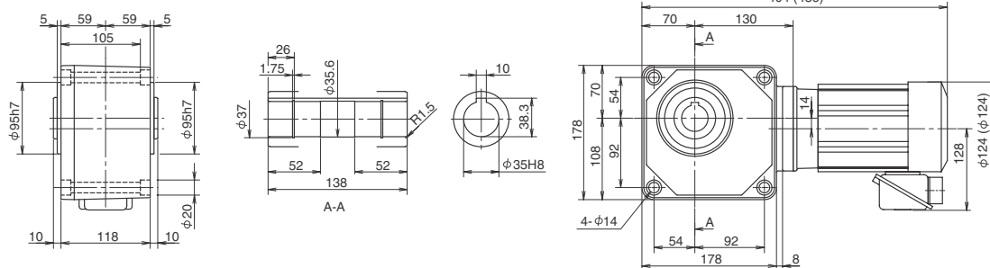
Fig. 5 RNYM03-1540-300~1440 Mass 26kg (RNYM03-1540-B-300~1440) (Mass 27.5kg)
