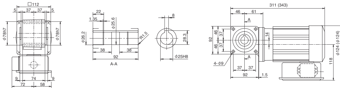
Fig. 2 RNYM02-1220-CB-5-30 (RNYM02-1220-CB-B-5-30) Mass 9.5kg (Mass 11kg)
