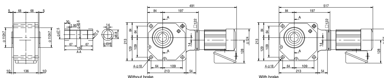
Fig. 5 RNYM03-1540-300~1440 Mass 26kg (RNYM03-1540-B-300~1440) (Mass 27.5kg)
