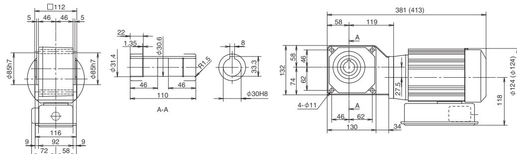
Fig. 3 RNYM02-1320-CB-40-60 (RNYM02-1320-CB-B-40-60) Mass 11kg (Mass 13kg)
