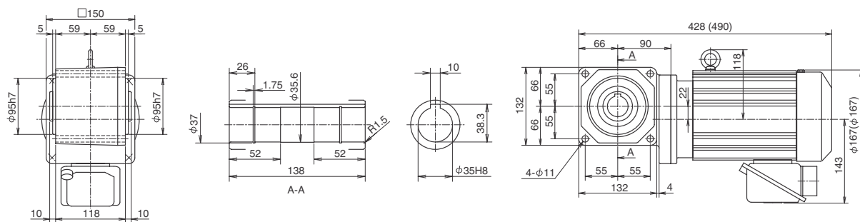
Fig. 2 RNYM1H-1420-5~30 (RNYM1H-1420-B-5~30) Mass 21kg (Mass 25kg)
