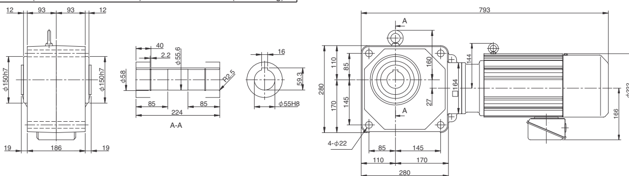
Fig. 2 RNYM8-1633-20~40 (RNYM8-1633-B-20~40)
