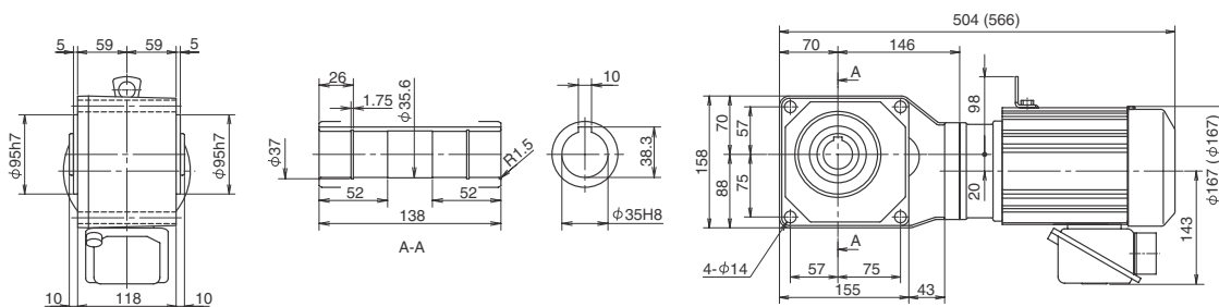
Fig. 2 RNYM1H-1420-5~30 (RNYM1H-1420-B-5~30) Mass 21kg (Mass 25kg)
