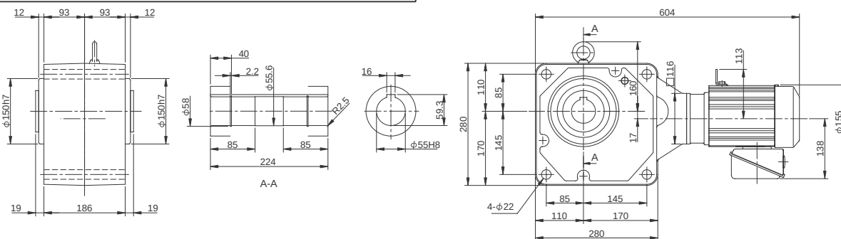
Fig. 5 RNYM05-1640-CB-300-1440 Mass 68kg (RNYM05-1640-CB-B-300-1440) (Mass 70kg)
