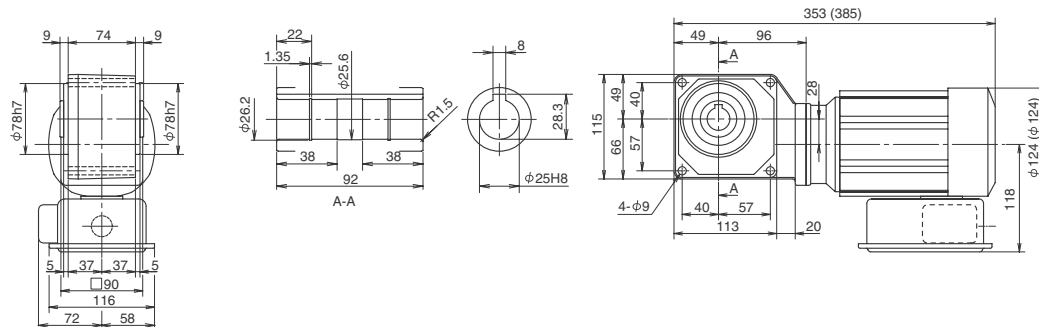
Fig. 2 RNYM02-1220-CB-5-30 (RNYM02-1220-CB-B-5-30) Mass 9.5kg (Mass 11kg)
