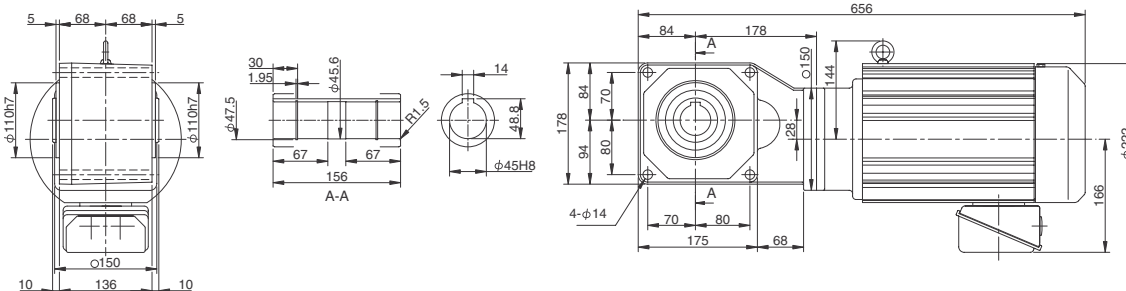
Fig. 2 RNYM8-1633-20~40 (RNYM8-1633-B-20~40)
