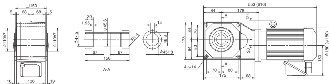
Fig. 2 RNYM3-1520-5~30 (RNYM3-1520-B-5~30) Mass 34kg (Mass 39kg)
